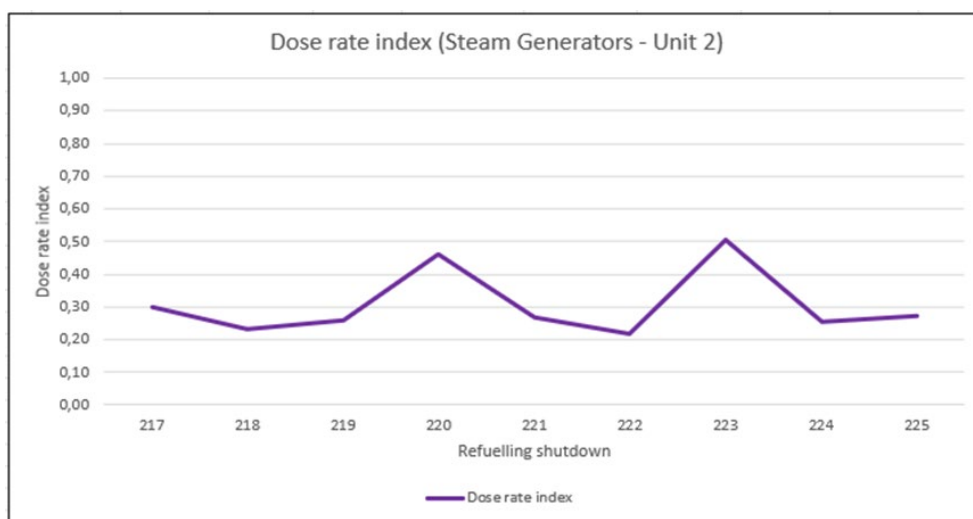
Figuur 20: Dosistempo-indeks vir Eenheid 2-stoomontwikkelaars
