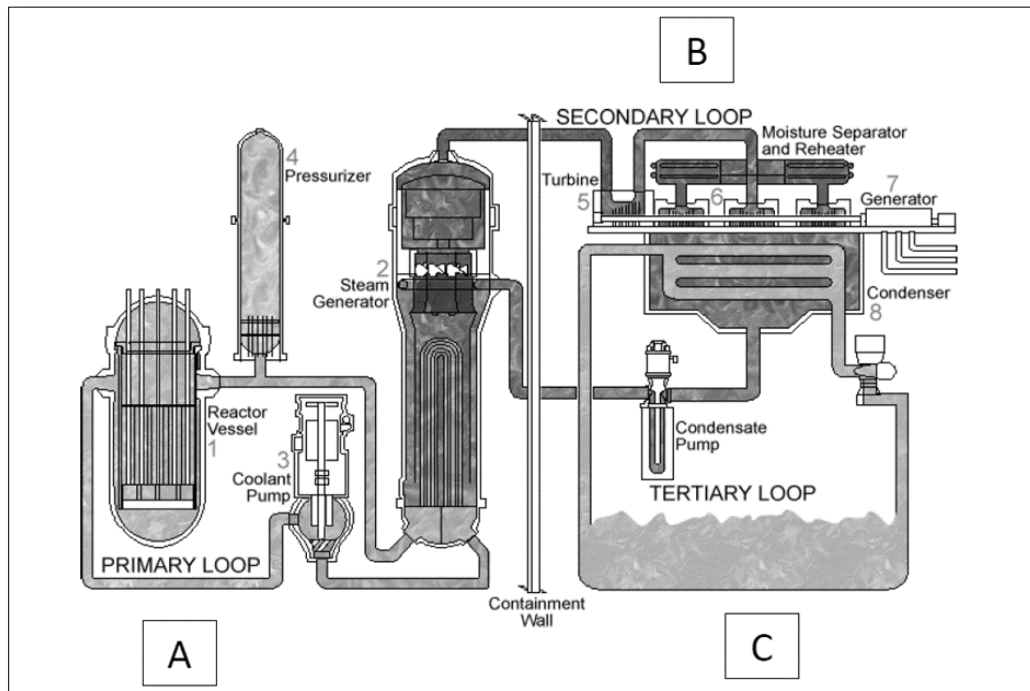
Figuur 6: Konfigurasie van stelsels van 'n PWR-aanlegontwerp [22]
