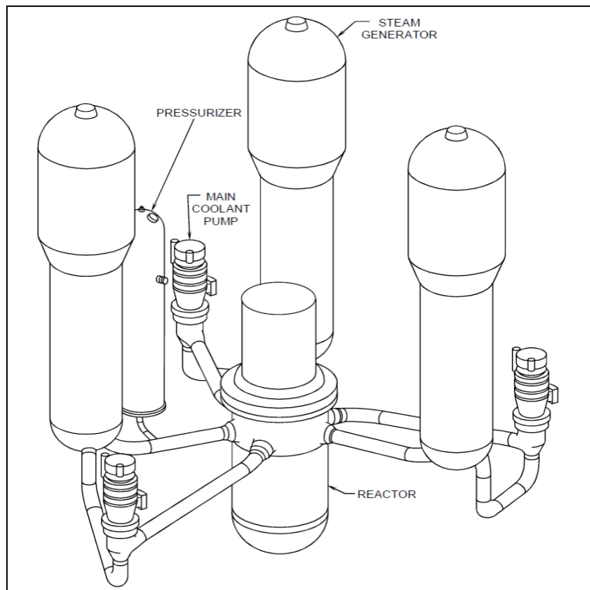
Figuur 7: Illustrasie van die algemene rangskikking van SSK's in 'n drieluskerkragaanleg [23]
