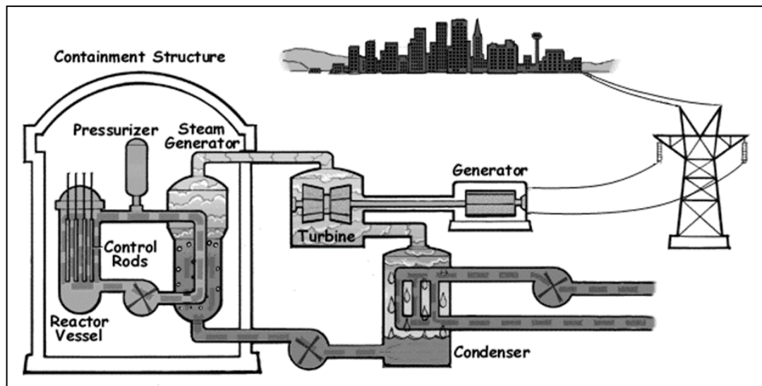
Figuur 5: Skematiese voorstelling van 'n tipiese drukwaterreaktor keraanleg [21]
