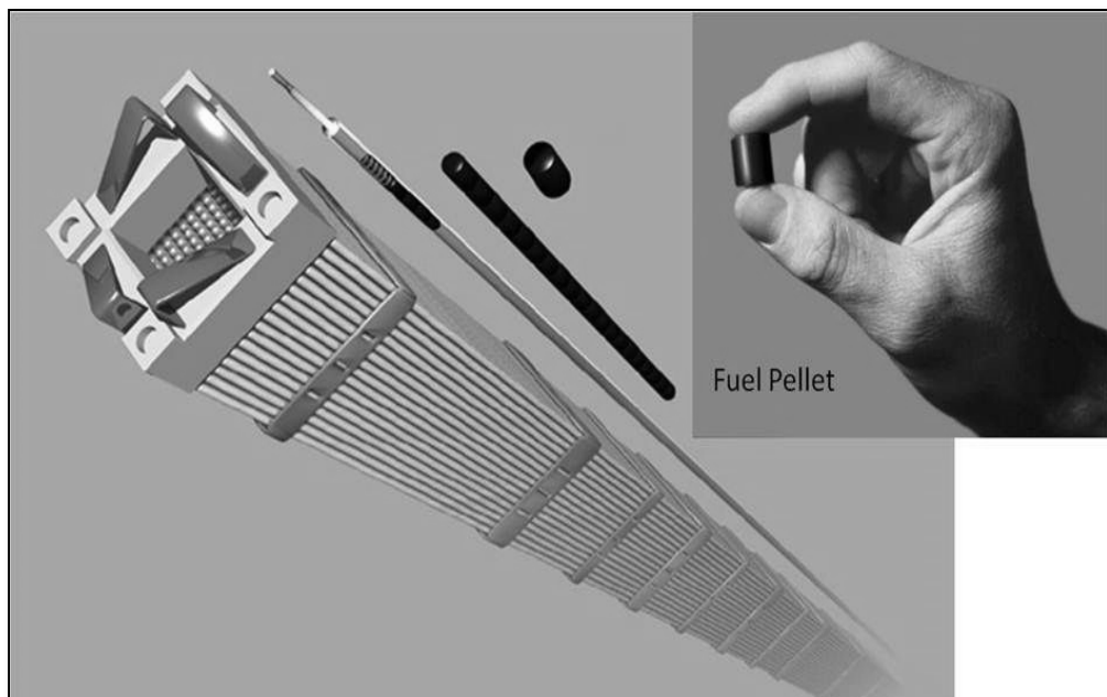
Figuur 9: Illustrasie van 'n tipiese PWR-kernbrandstofelement, met die brandstofstaaf, beheerstaaf, en brandstofpillelemente afsonderlik getoon
