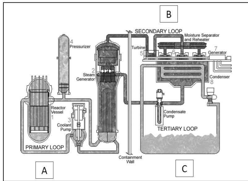
Figuur 6: Konfigurasie van stelsels van 'n PWR-aanlegontwerp [22]
