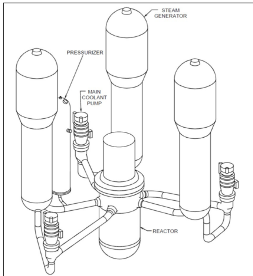
Figure 7: Illustrasie van die algemene rangskikking van SSK's in 'n drieluskernkragaanleg [23]
