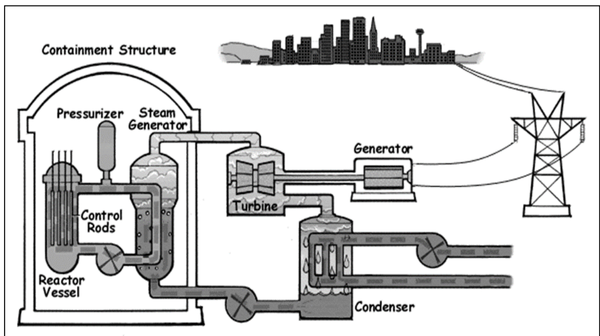
Figuur 5: Skematiese voorstelling van 'n tipiese drukwaterreaktor kernaansleg [21]
